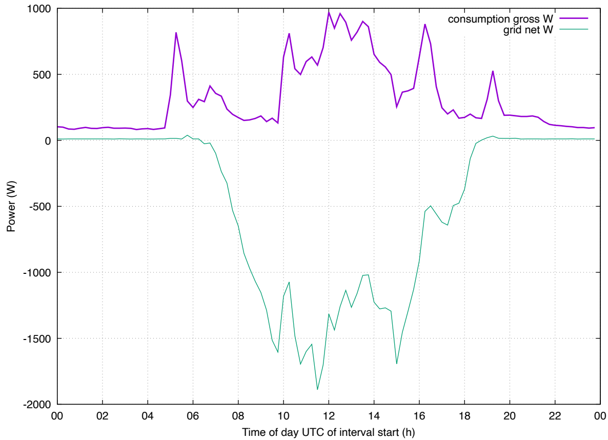
Load Profile: 202606 enphase all
