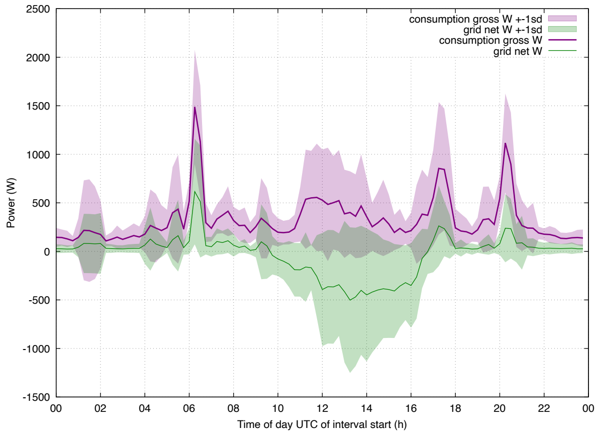
Load Profile: 202603 enphase all
