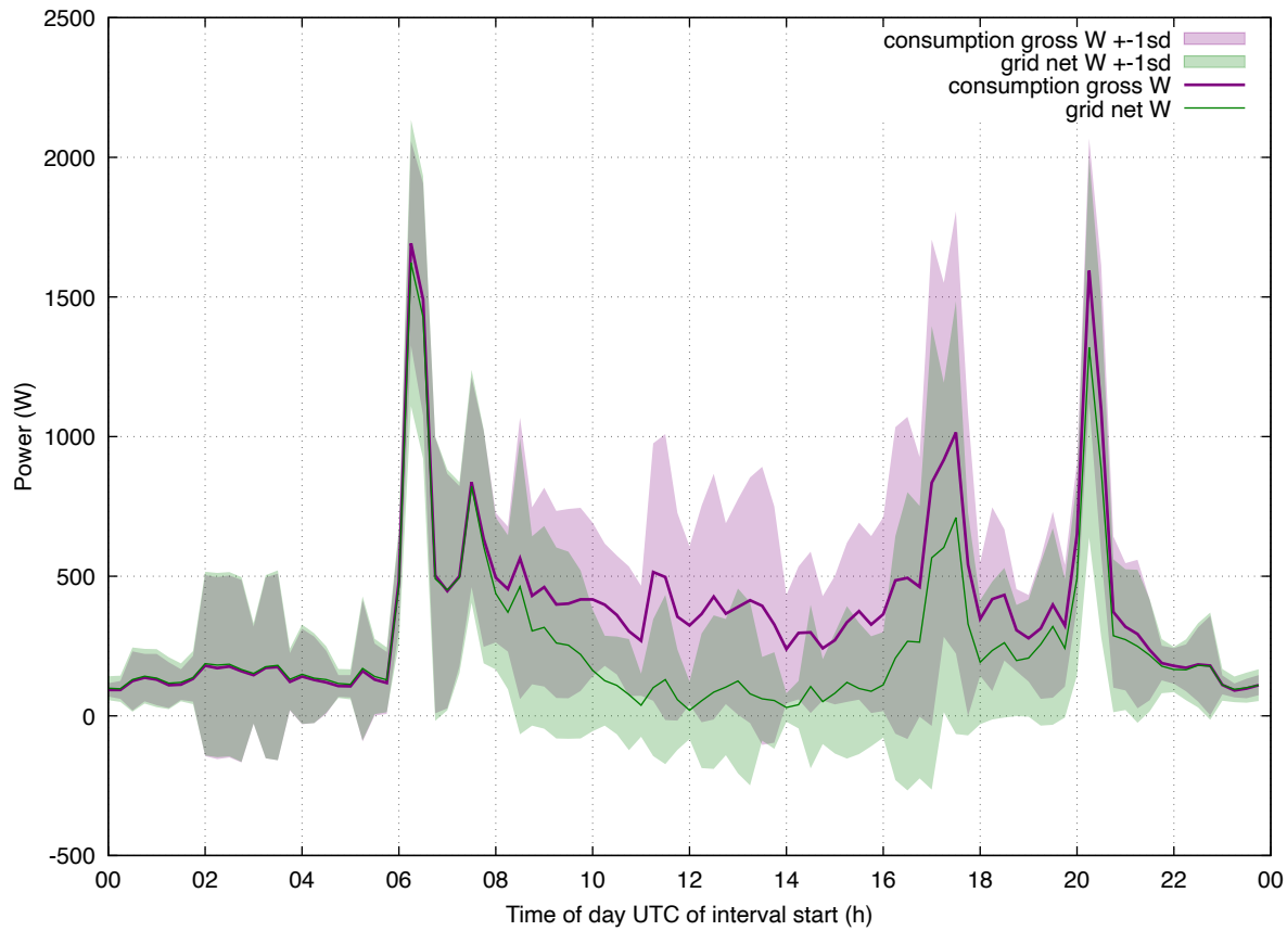
Load Profile: 202602 enphase all
