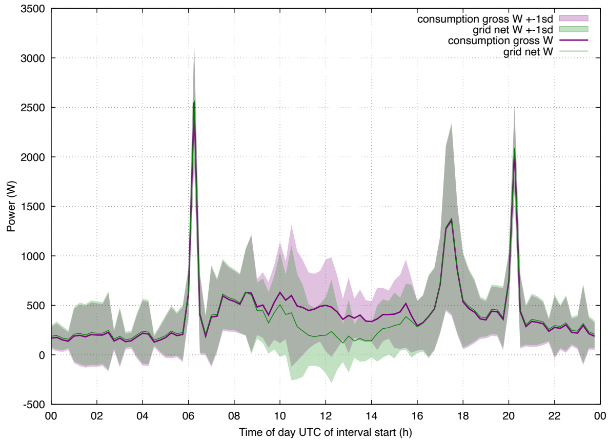
Load Profile: 202512 enphase all
